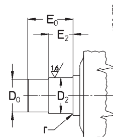
e) Perno macchina «corto» e) «Short» shaft end of driven machine
