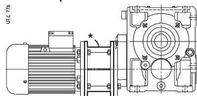
MLS / MLA montaggio tra riduttore e motore o motovariatore mounted between gear reducer and motor or motor-variator
