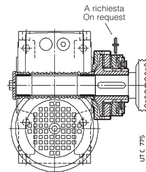
Montaggio limitatore intermedio Intermediate limiter mounting
